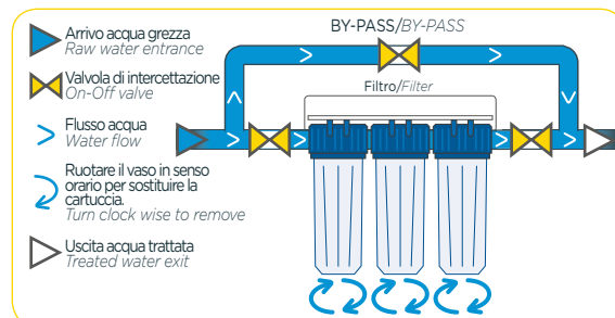
N.B.: Schema di installazione completo a pag.49/Complete installation scheme p.49
